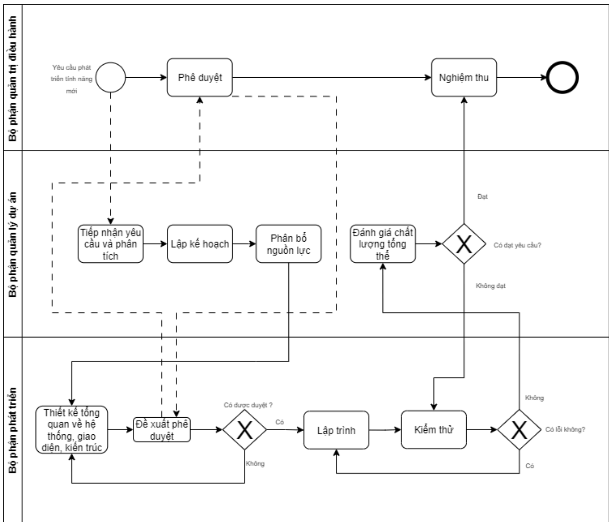
Hình 3.6. Mô hình BPMN phát triển tính năng mới.
