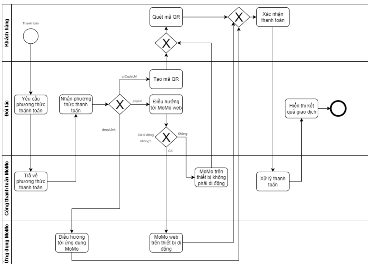
Hình 3.8. Mô hình BPMN quy trình thanh toán.
