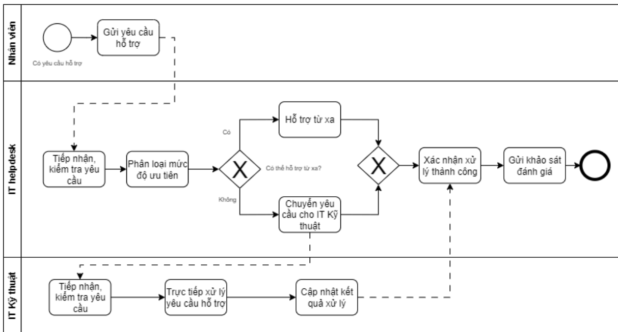
Hình 3.12. Mô hình BPMN quy trình hỗ trợ nội bộ.
